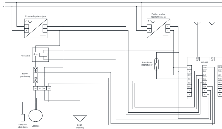
Rys.2.Przykładowy schemat połączeń MT-652 w SOK.
